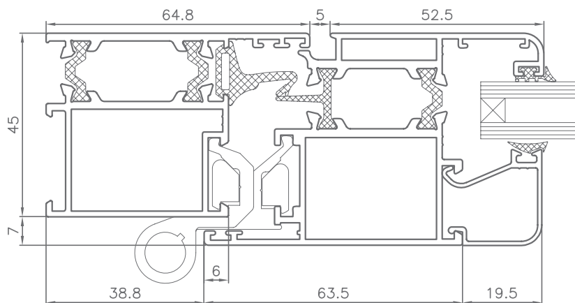
NUDO LATERAL PERFIL DE PUERTA
